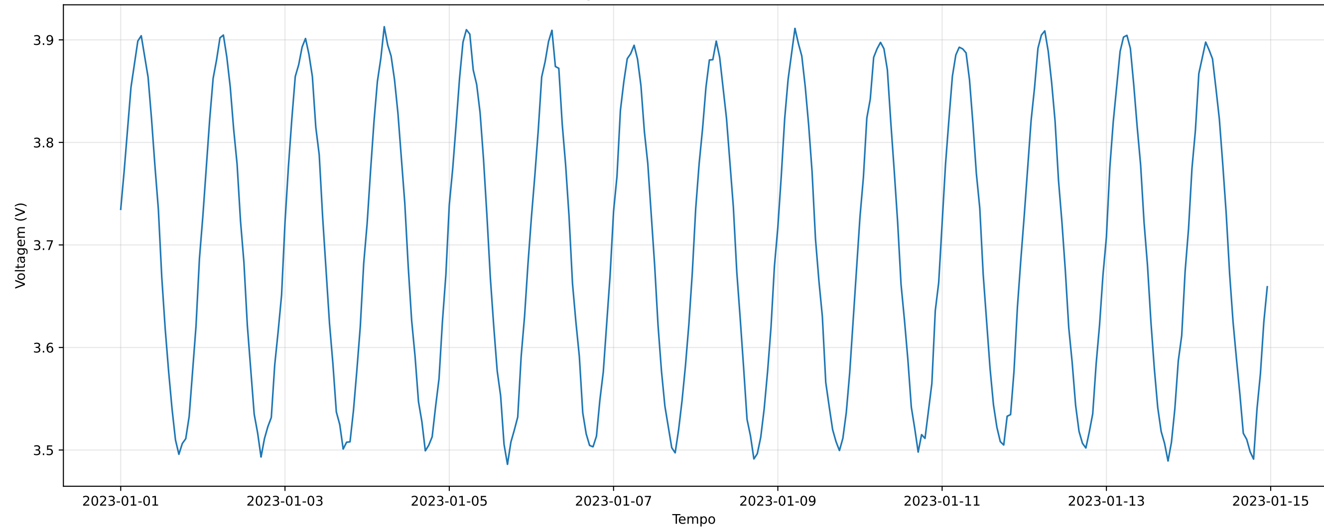
Voltagem da bateria — média horária
